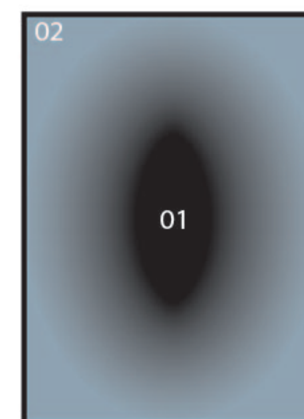
Nimbus
