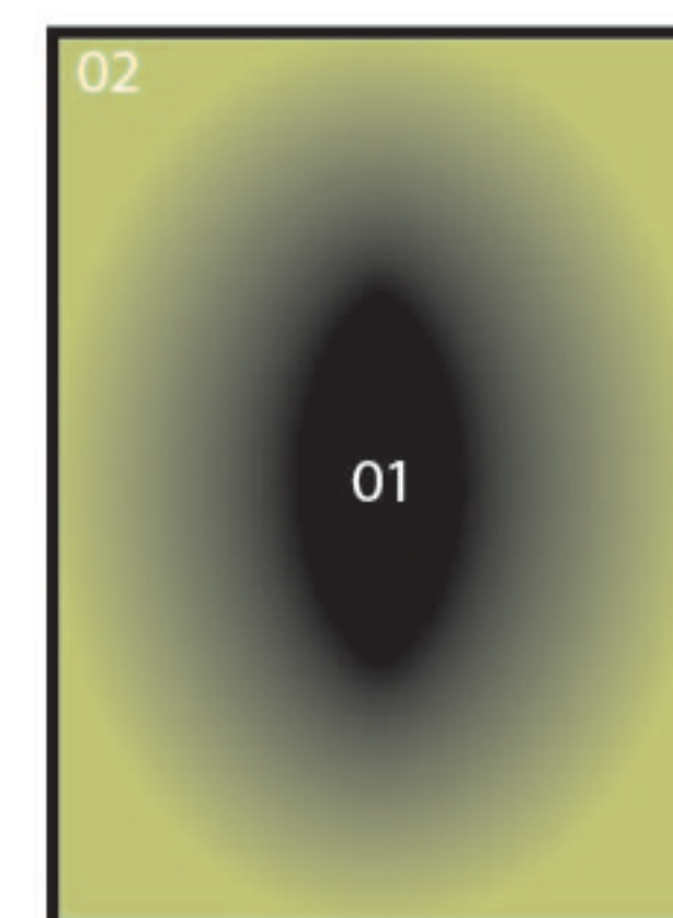
Nimbus
