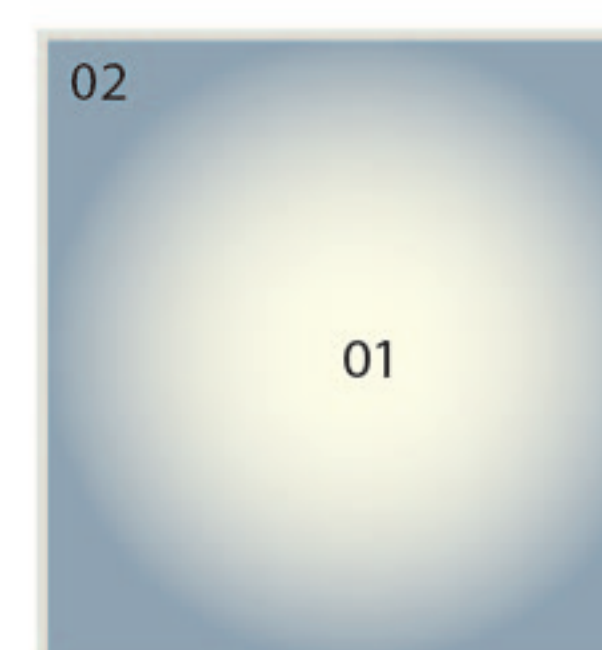
Cirrus
