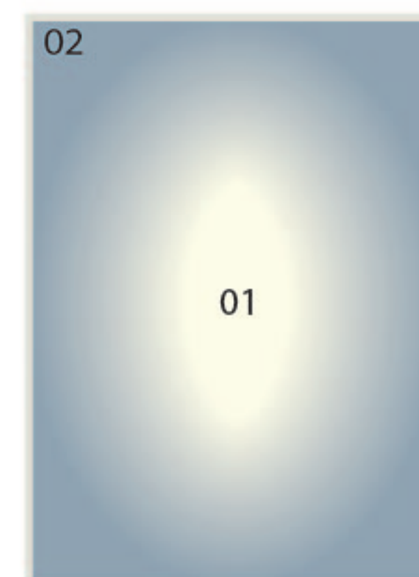
Nimbus
