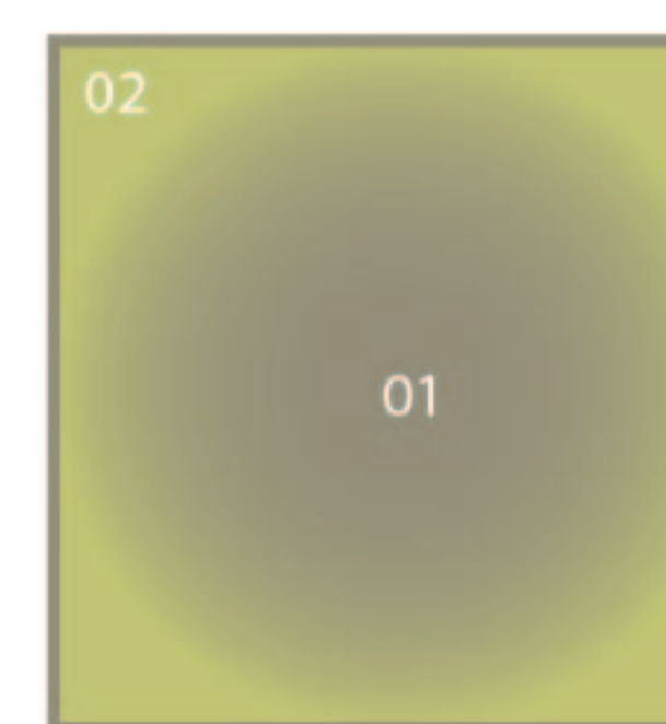
Cirrus
