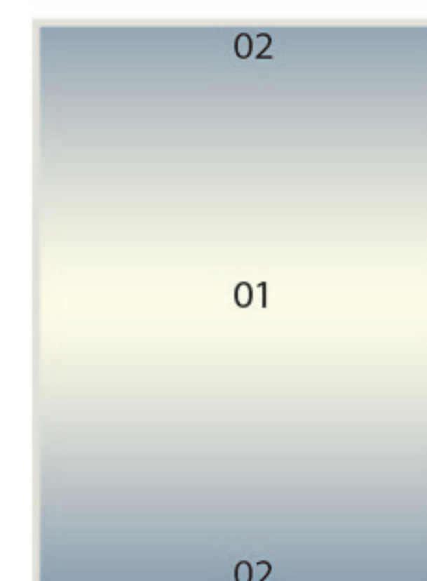
Cumulus
