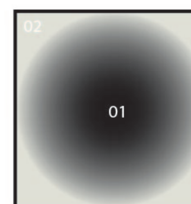
Cirrus
