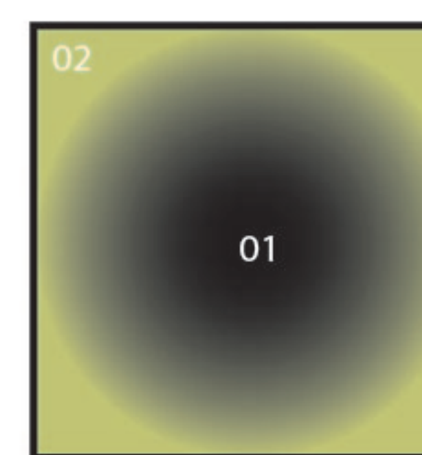
Cirrus
