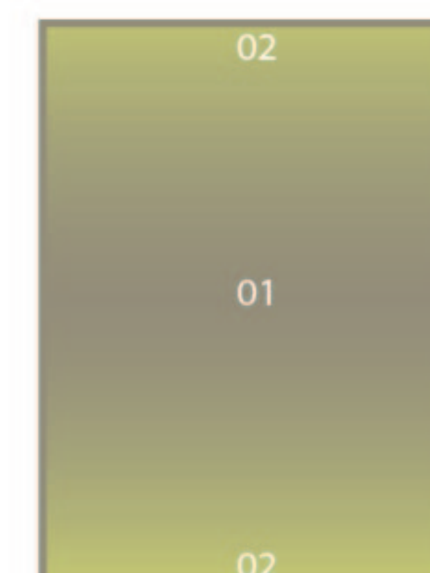
Cumulus
