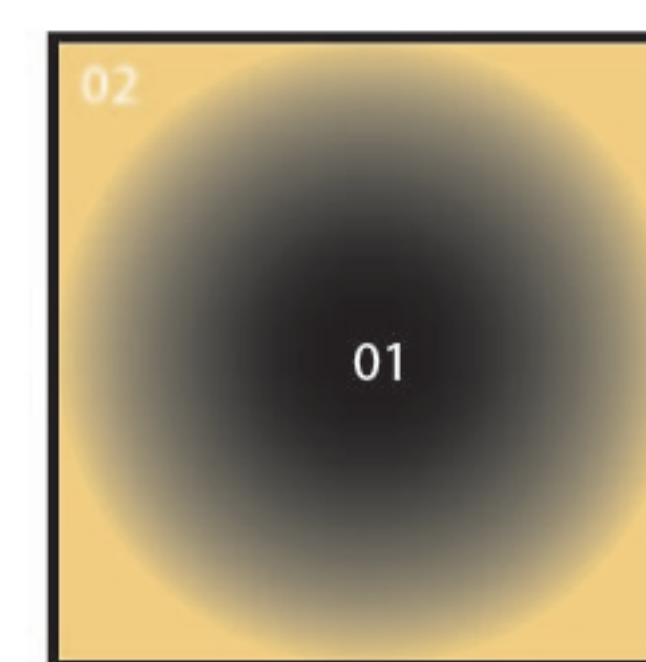
Cirrus
