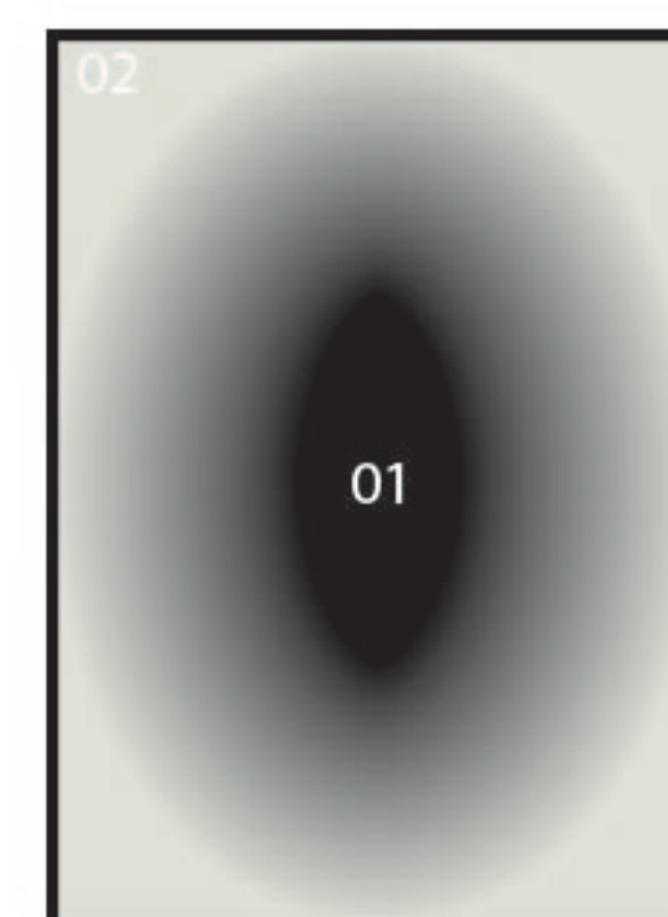
Nimbus
