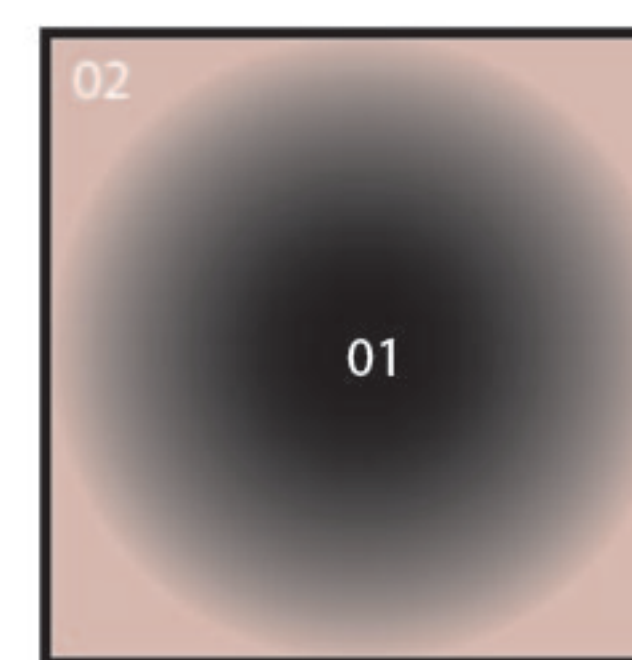
Cirrus
