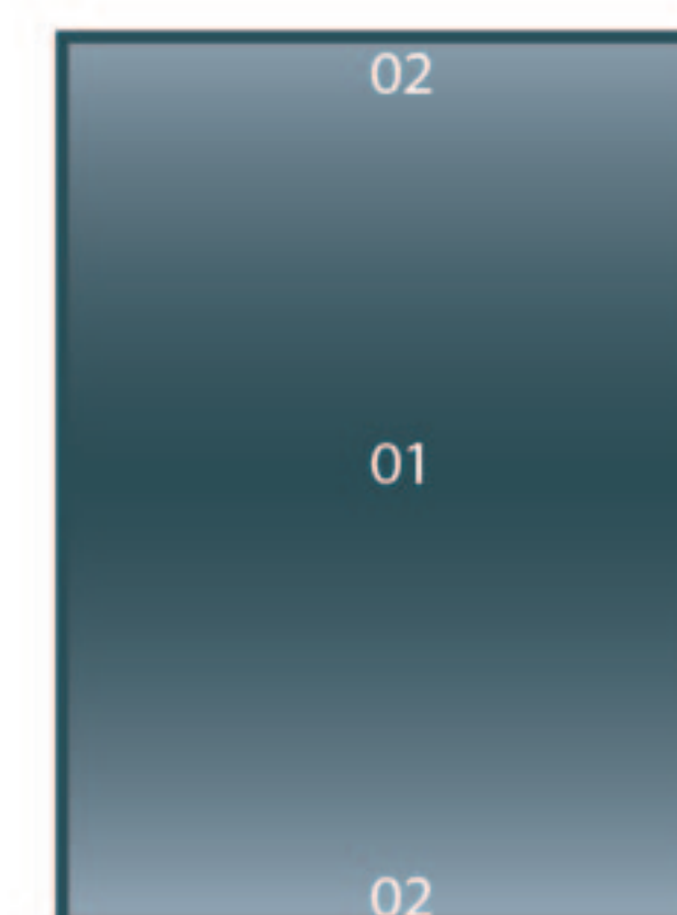
Cumulus
